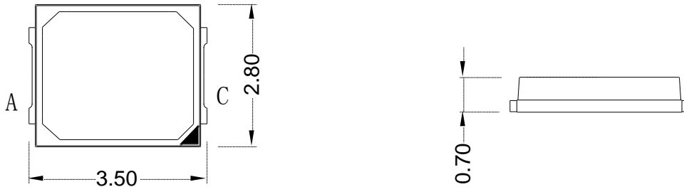
Fig.1-1 Top view 正面视图 Fig.1-2 Side view 侧面视图
