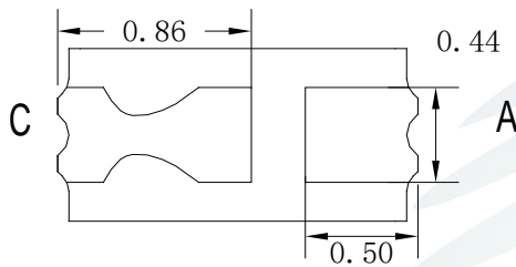
Fig. 1-3 Bottom View 背面视图
