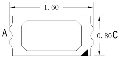
Fig. 1-1 Top View 正面视图
