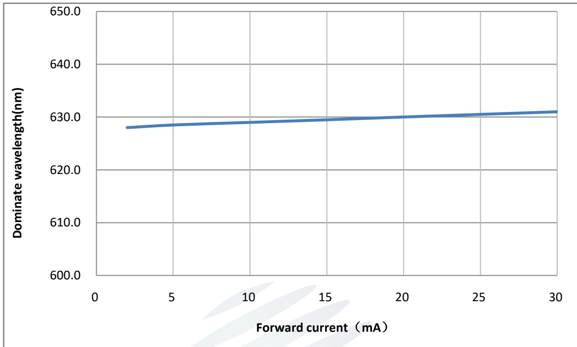
Fig. 1-13 Forward Current vs. Color Shift (Ts=25°C)正向电流与主波长特性曲线 (Ts=25°C)
