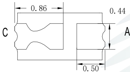
Fig. 1-3 Bottom View 背面视图
