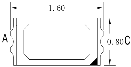
Fig. 1-1 Top View 正面视图
