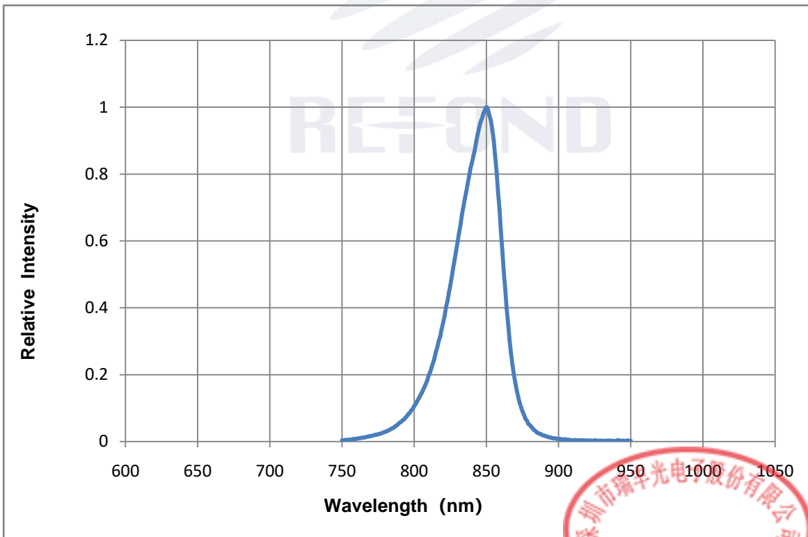
Fig. 1-14 Spectrum Distribution光谱分布特性曲线
