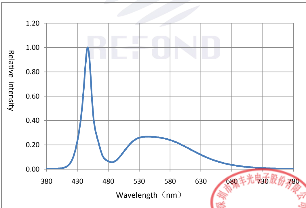
Fig. 1-14 Spectrum Distribution光譜分布特性曲线
