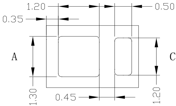
Fig.1-3 Bottom View 背面视图
