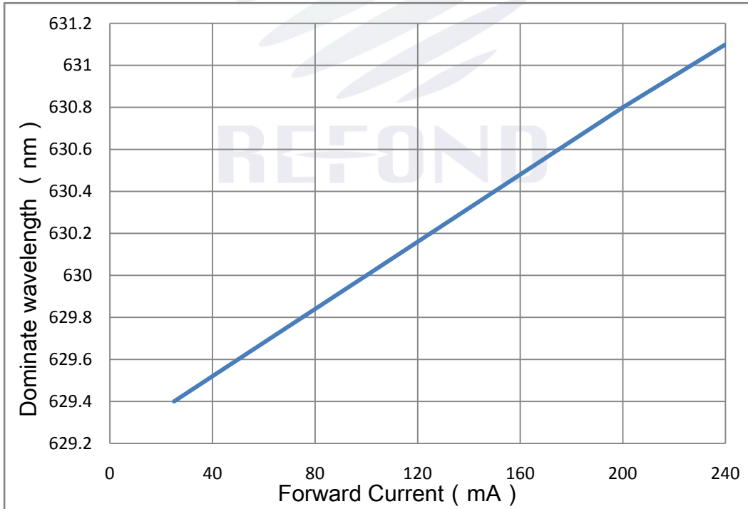
Fig. 1-12 Forward current vs. Color Shift 正向电流与主波长特性曲线 (Ts=25°C)
