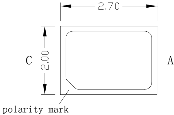
Fig.1-1 Top View 正面视图
