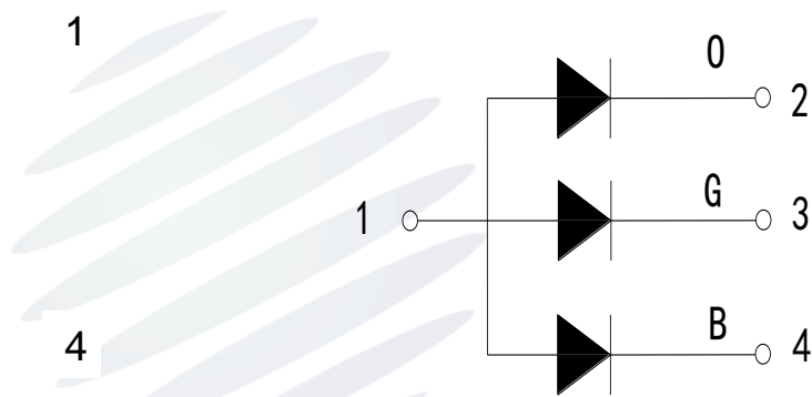
Fig.1-4 Polarity 极性
