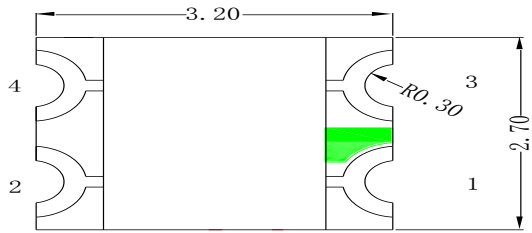
Fig.1-1 Top view 正面视图
