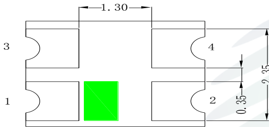
Fig.1-3 Bottom view 背面视图
